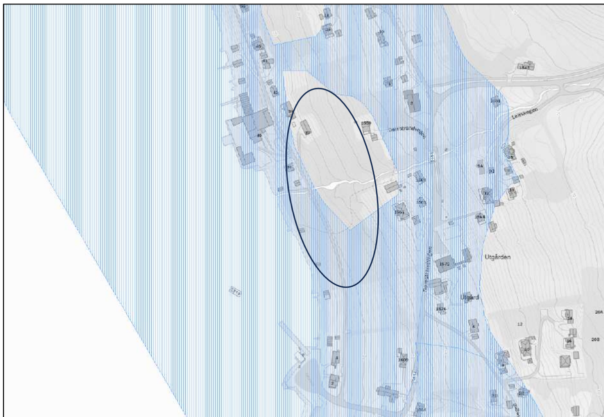
Figur 7 Atksomhetssone for marin leire
