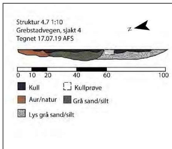
Figur 32 Struktur 4.7 i profil.
