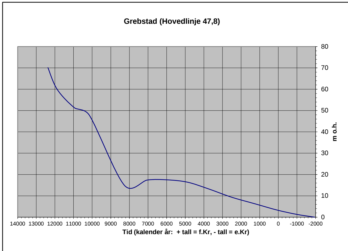
Figur 6: Strandlinjekurve for Grebstad i Sykkylven kommune etter skjema utarbeidet av David N. Simpson, mars 2001 (jfr. Svendsen & Mangerud 1987, Bondevik, Svendsen og Mangerud 1998).
