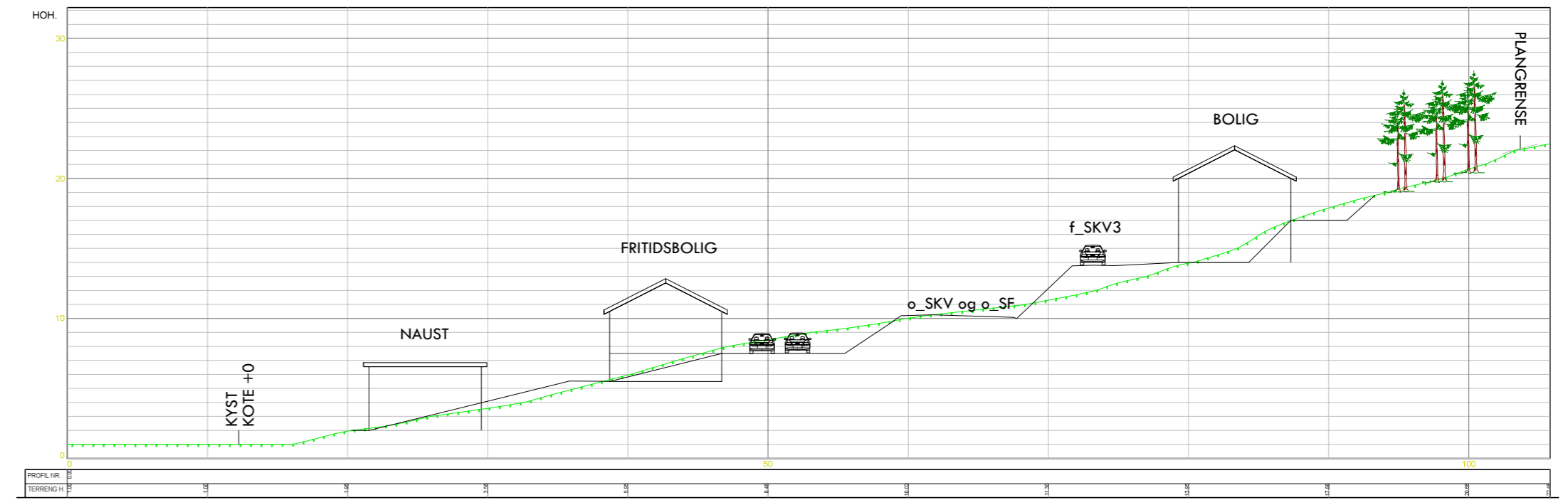
SNITT 2
