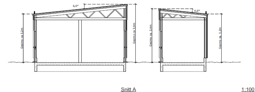
Figur 21 Snitt av boder. Kilde: Norgeshus AS.
