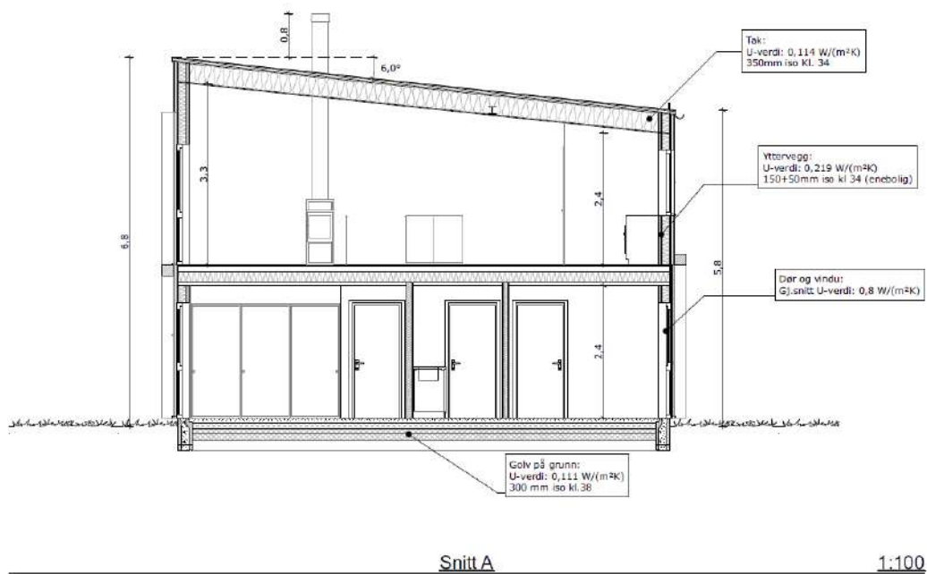
Figur 20 Snitt av tomannsboliger. Kilde: Norgeshus AS.
