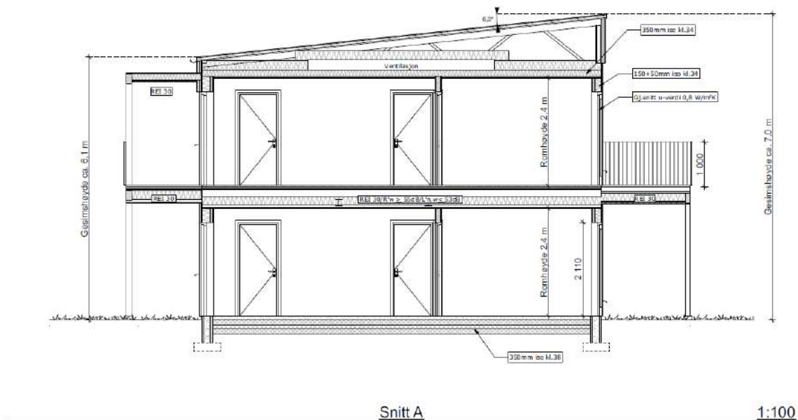
Figur 19 Snitt av seksmannsboliger. Kilde: Norgeshus AS.
