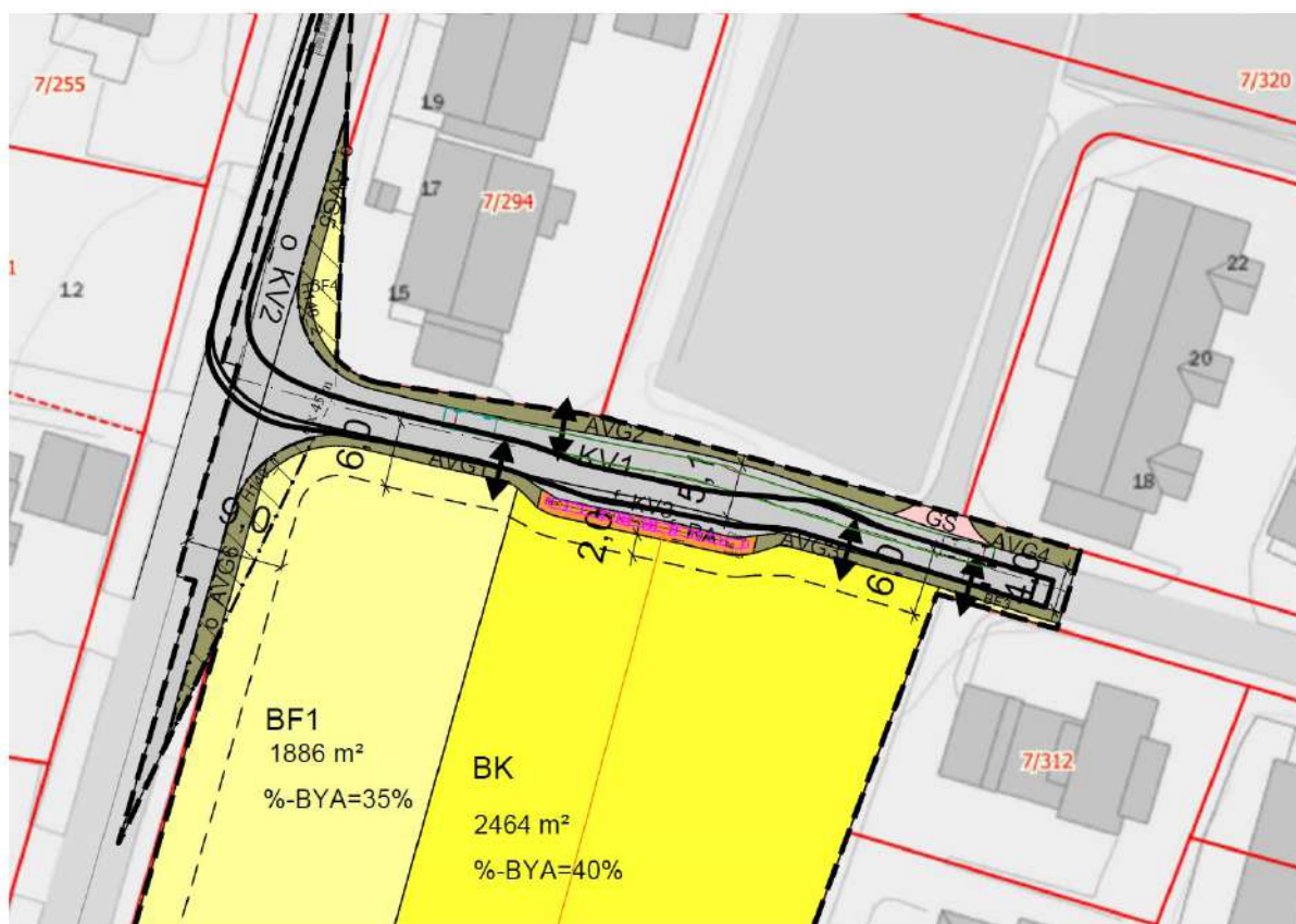
Figur 24 Hentepunkt med sporingskurver.
