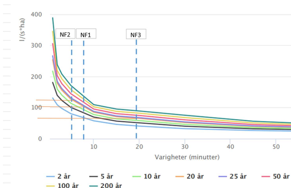
Figur 3: IVF-kurve for Ålesund – Spjelkavik (SN60940) med beregna verdier
